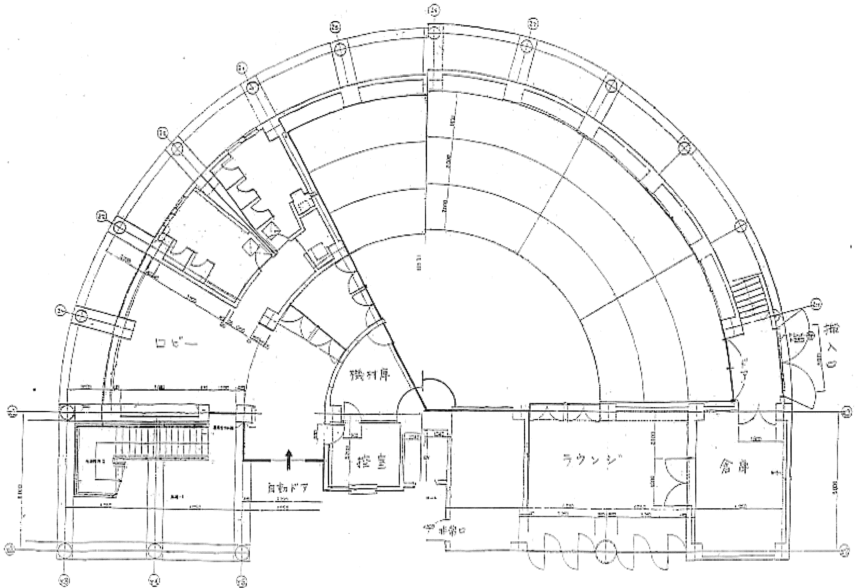
小ホール平面図
